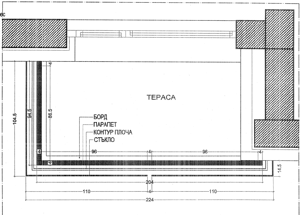
ДЕТАЙЛ - ПЛАН М 1:20
