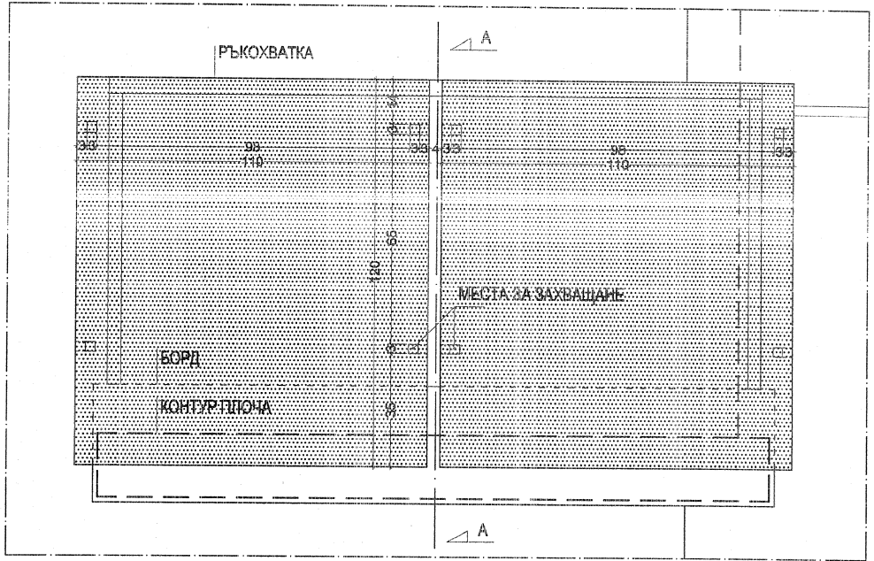
ДЕТАЙЛ - ИЗГЛЕД М 1:20
