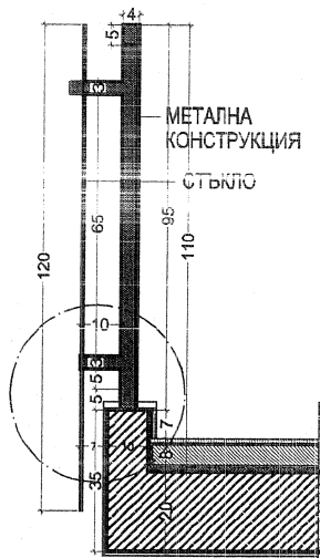
РАЗРЕЗ А-А М 1:20
